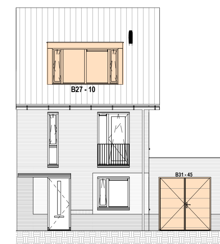
VOORGEVEL 1:100
