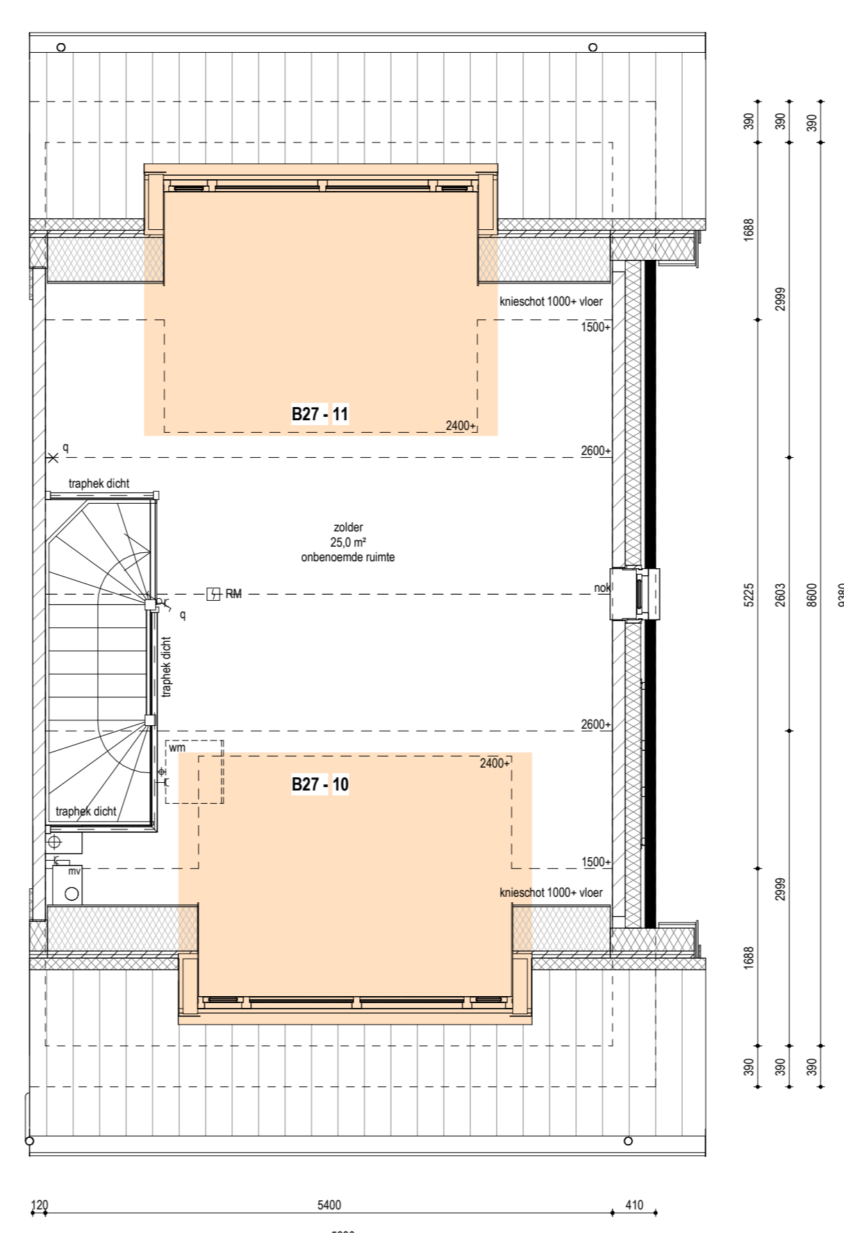
TWEDE VERDIEPING 1:50
