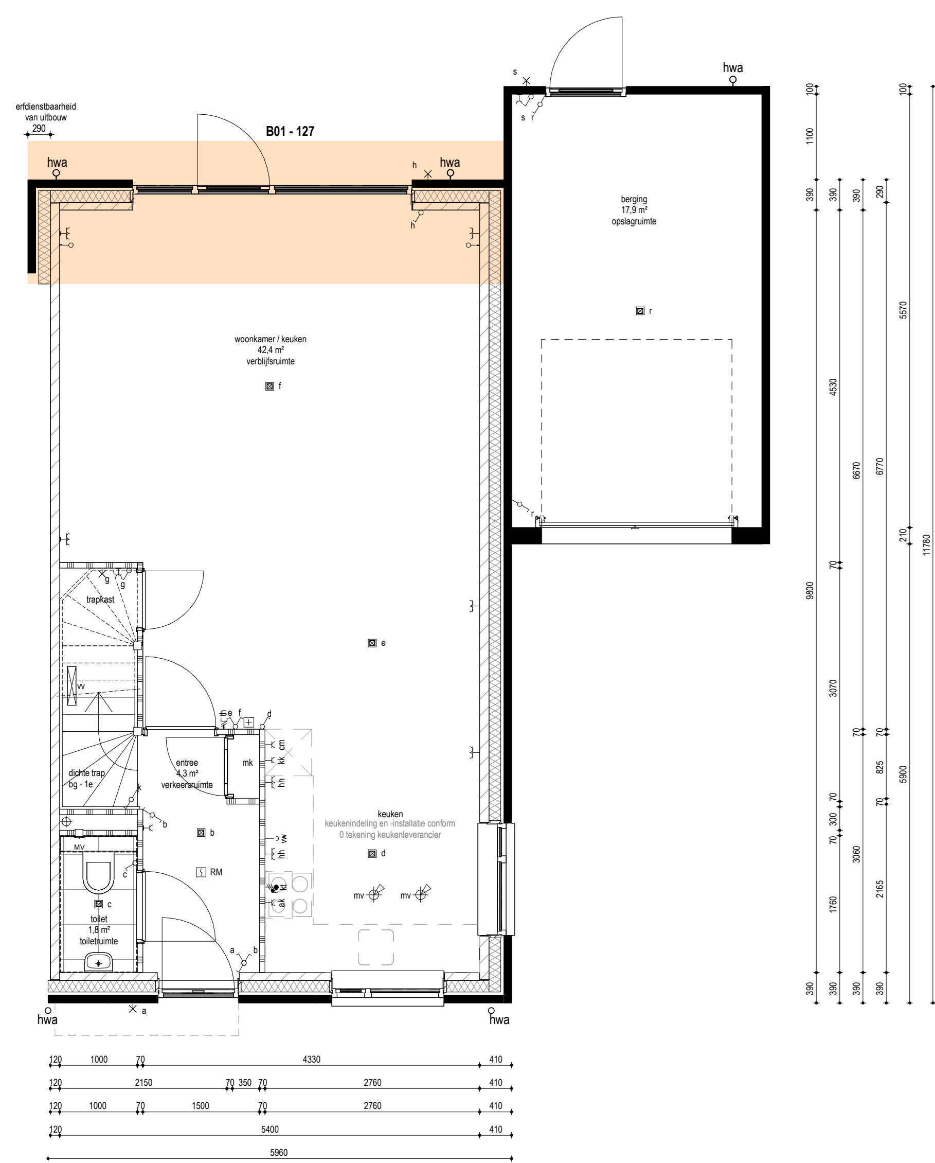
BEGANE GROND 1:50
