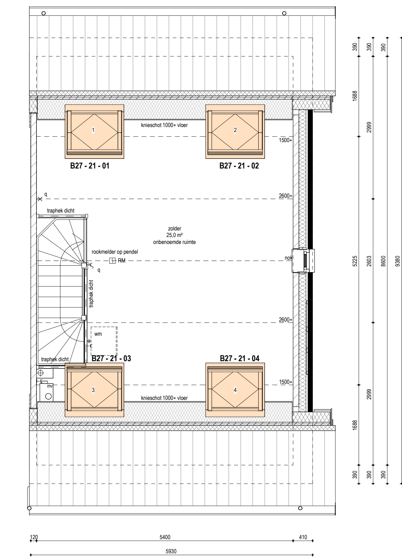
TWEDE VERDIEPING 1:50 optie dakramen bouwnummer 10
