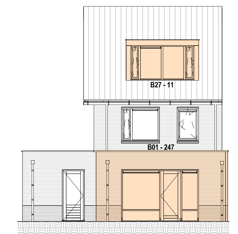
ACHTERGEVEL 1:100
