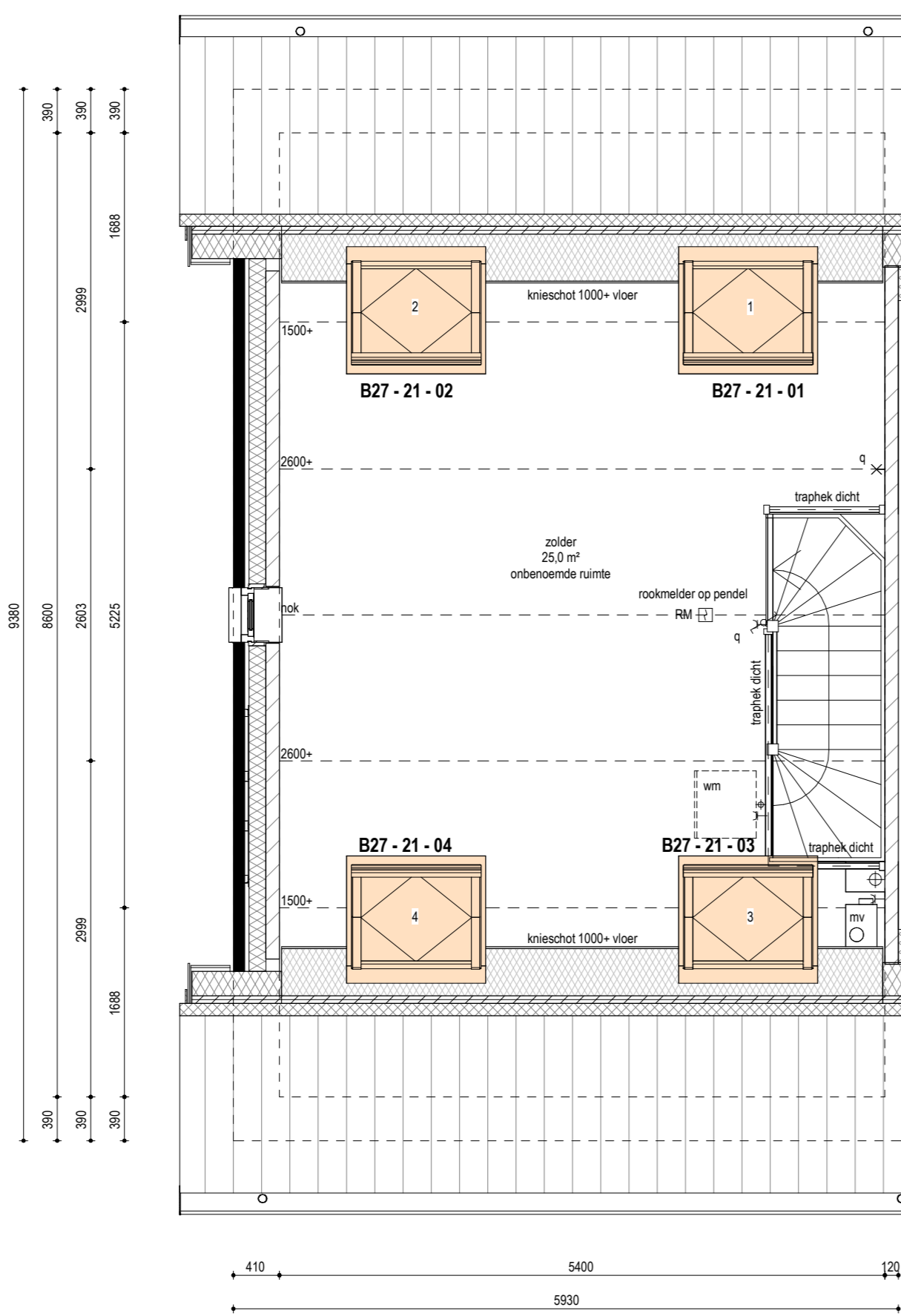
TWEDE VERDIEPING GESPIEGELD 1:50 optie dakramen bouwnummer 10
