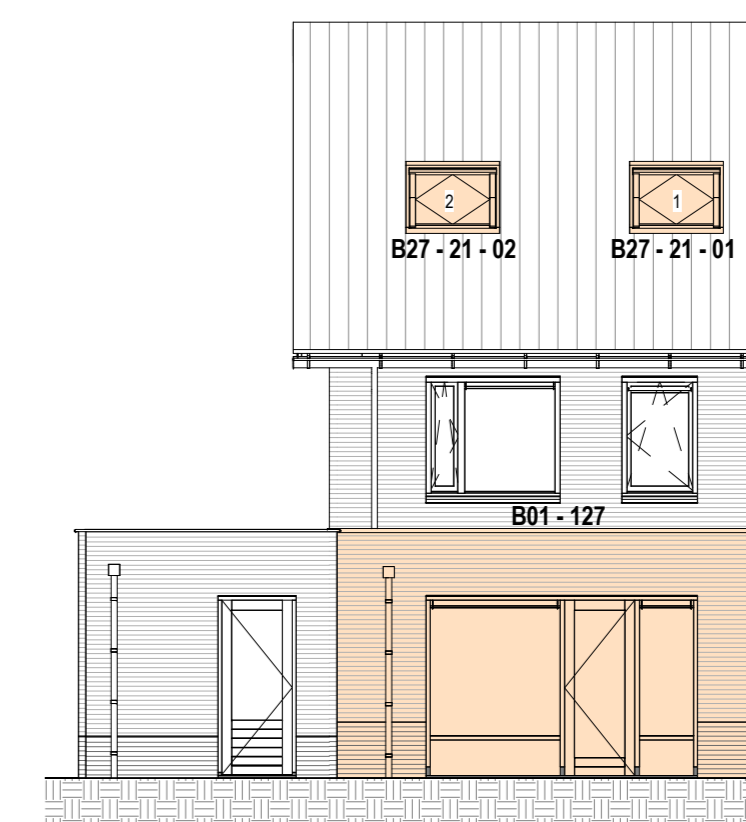
ACHTERGEVEL 1:100
