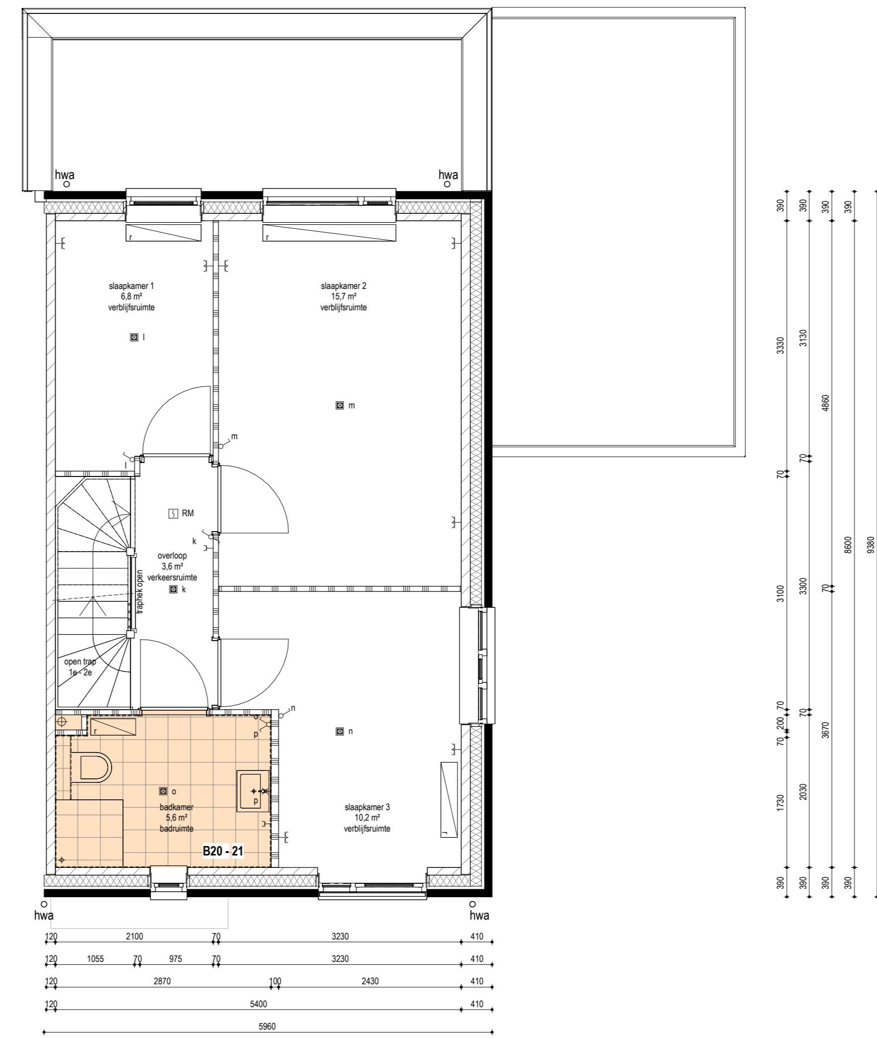
EERSTE VERDIEPING 1:50
