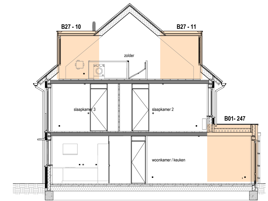
DOORSNEDE 1:100
