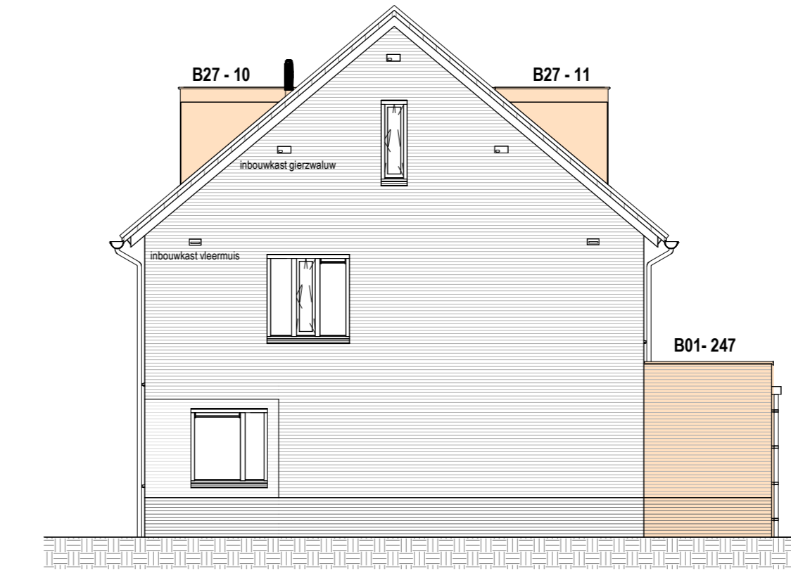
ZIJGEVEL 1:100
