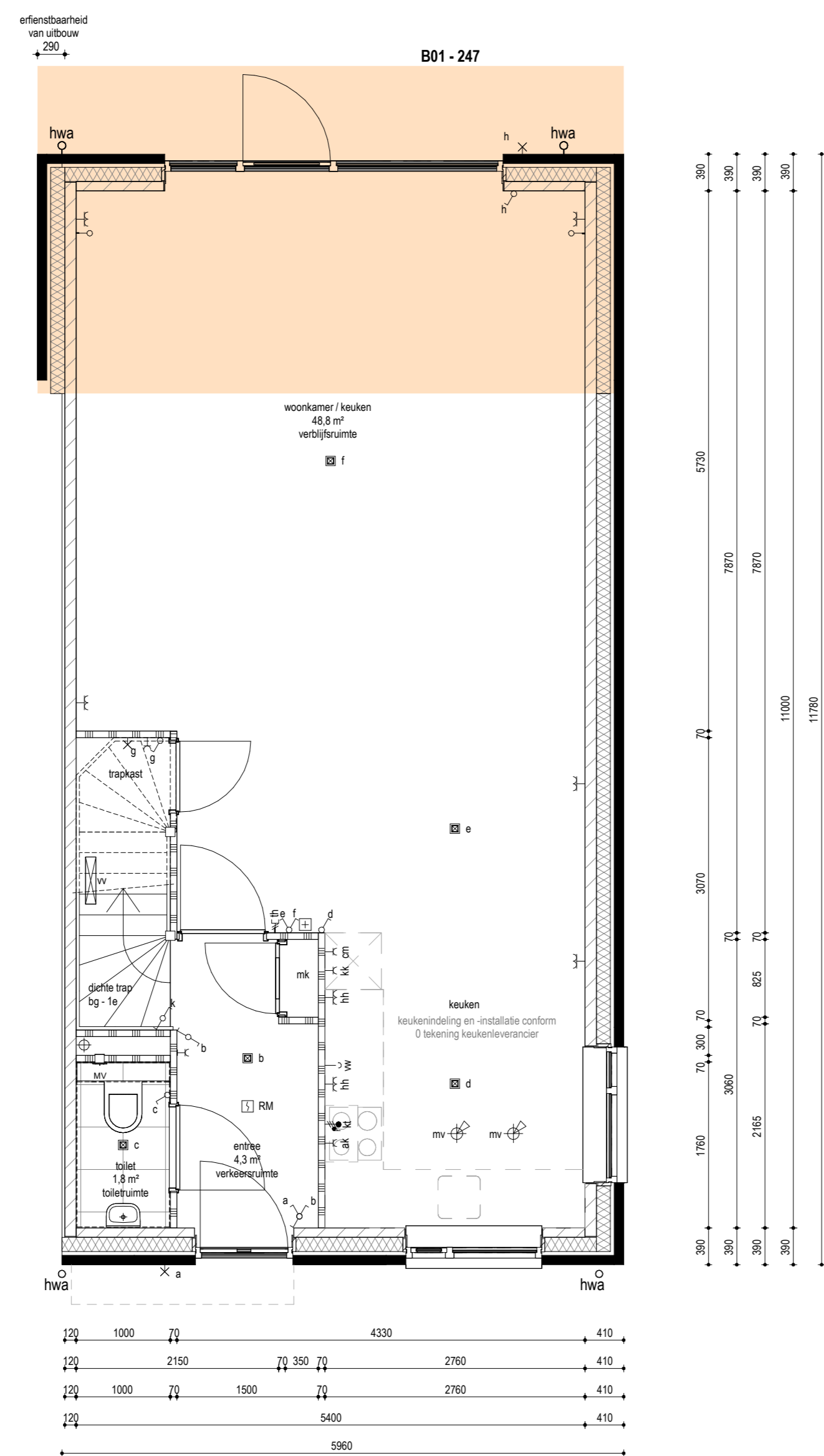
BEGANE GROND 1:50
