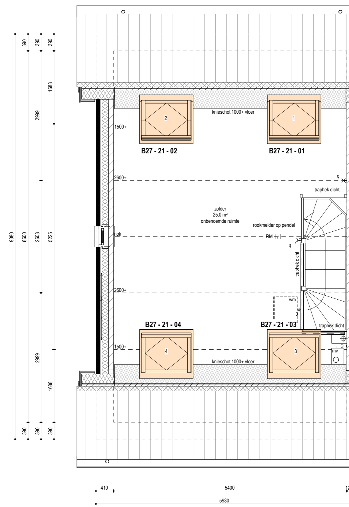
TWEDE VERDIEPING GESPIEGELD 1:50 optie dakramen bouwnummer 20
