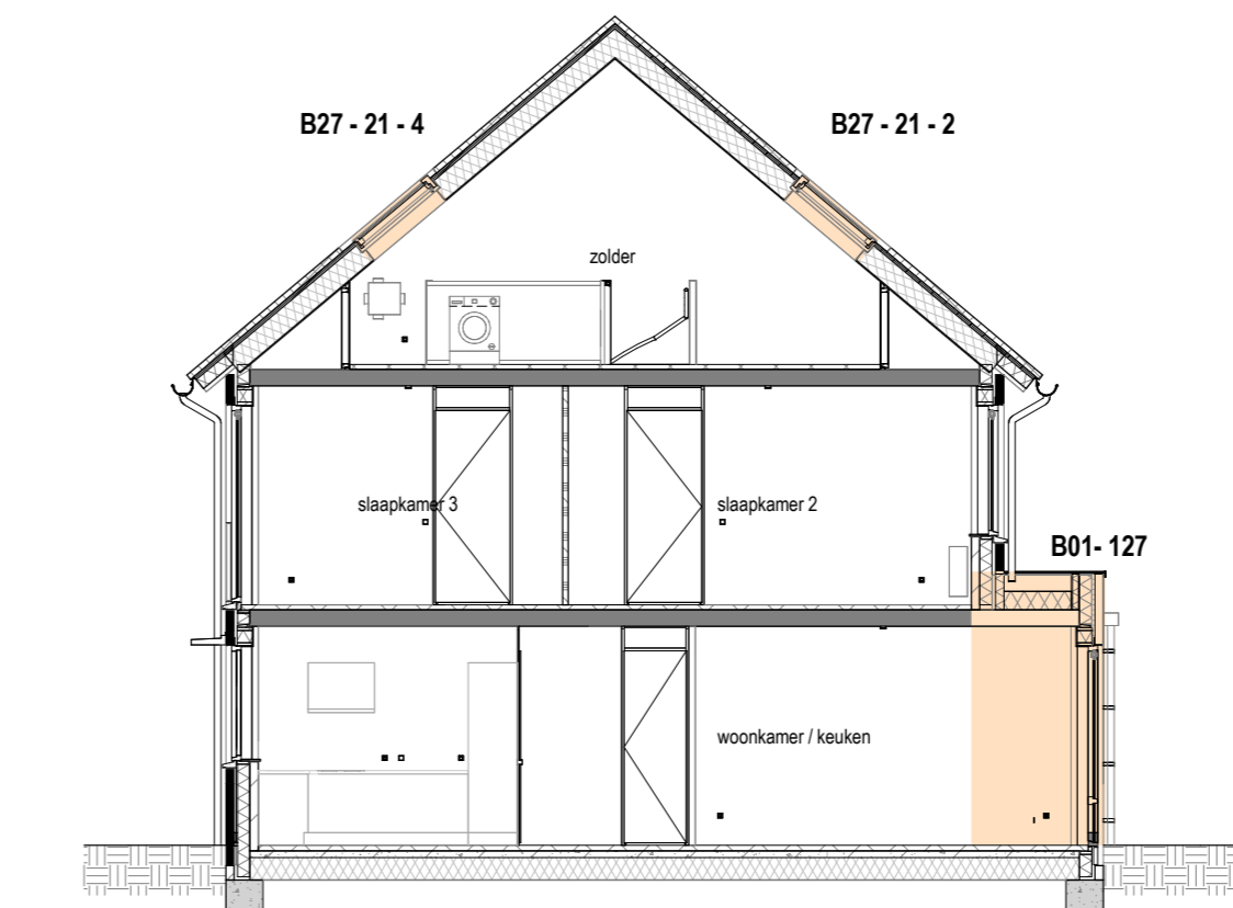
DOORSNEDE 1:100
