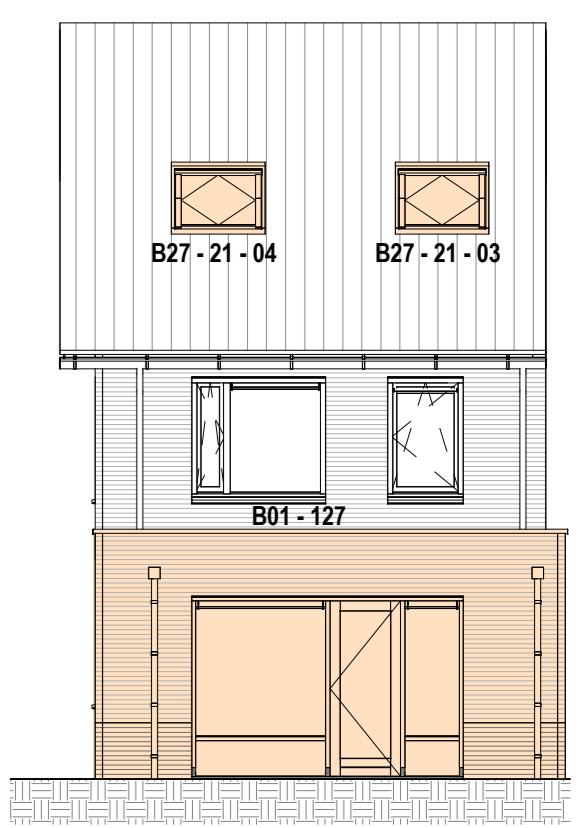
ACHTERGEVEL 1:100
