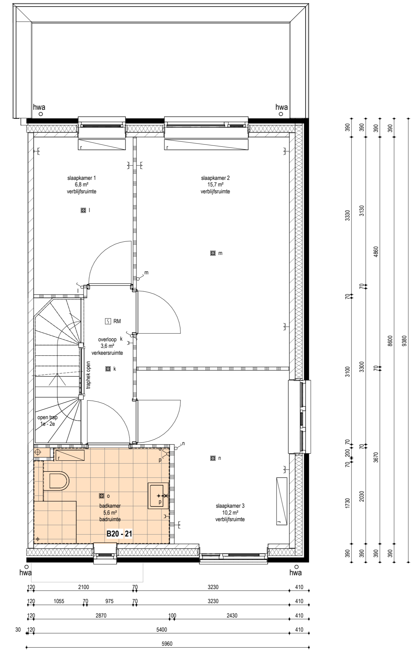
EERSTE VERDIEPING 1:50
