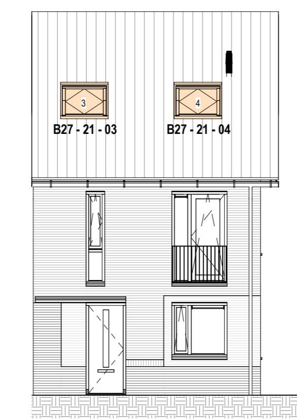
VOORGEVEL 1:100
