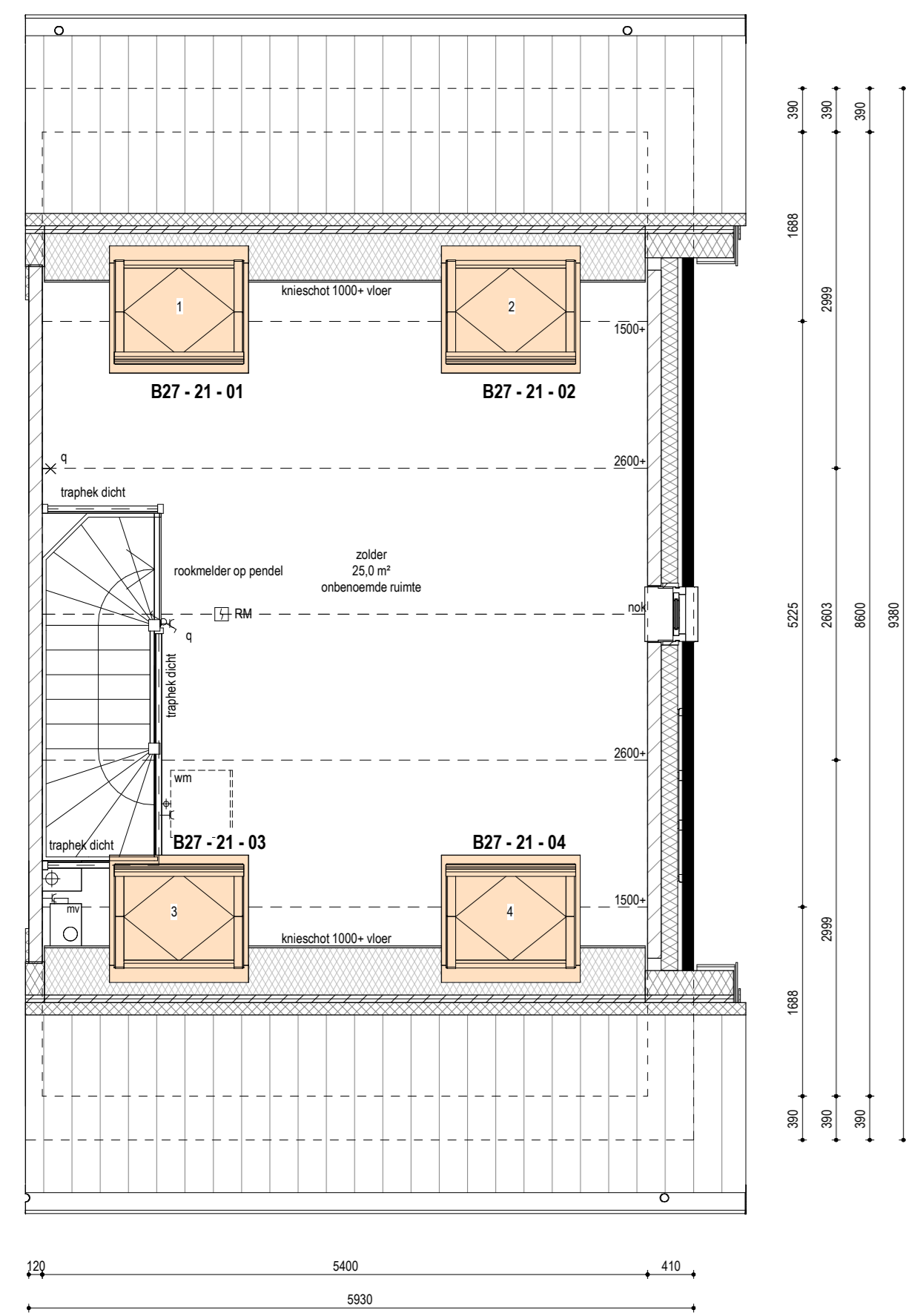
TWEDE VERDIEPING 1:50 optie dakramen bouwnummer 14
