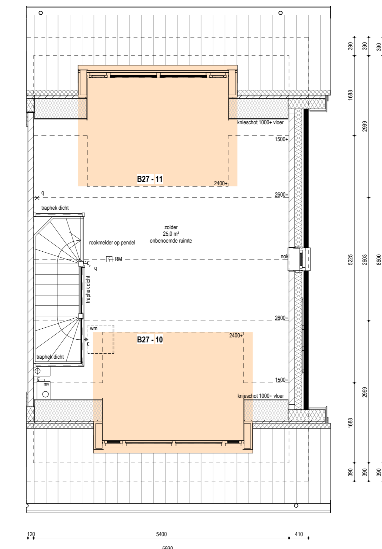
TWEDE VERDIEPING 1:50
