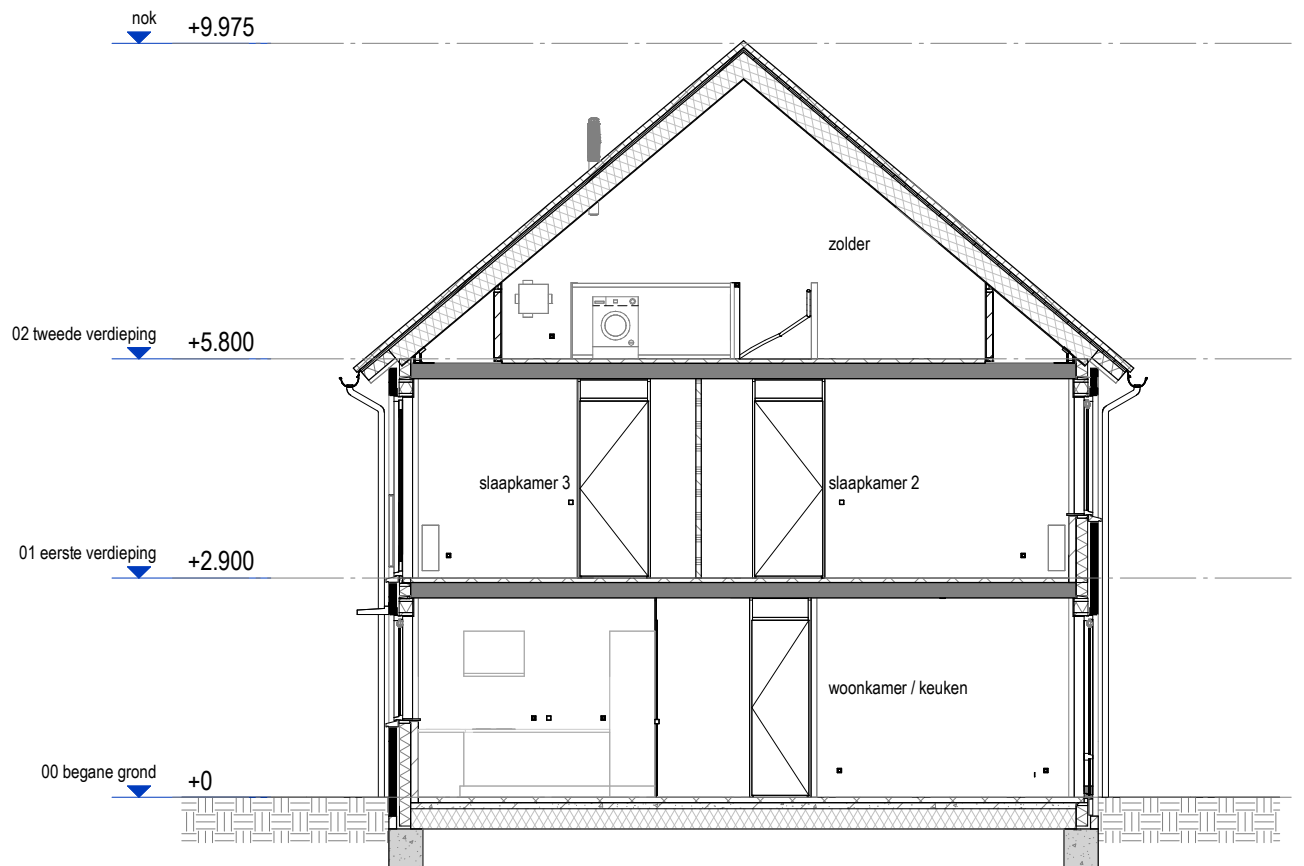
DOORSNEDE 1 : 100
